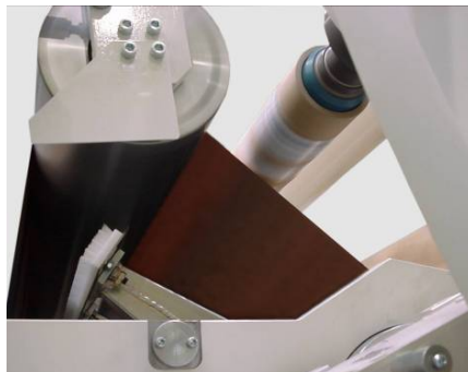
在切割前的TAC自动换卷系统
