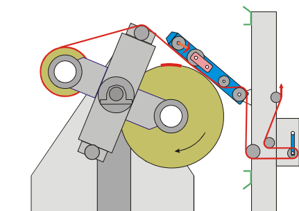
放卷机 UW 1500 S: 上部粘贴系统
