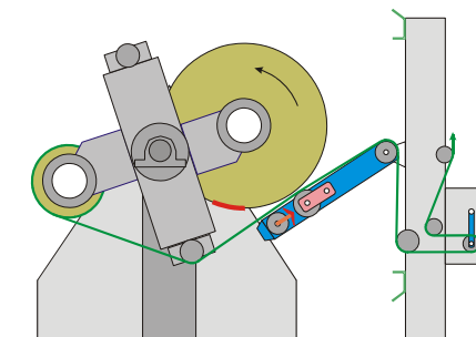
放卷机 UW 1500 S: 下部粘贴系统
