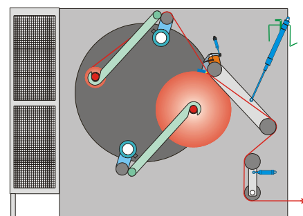
放卷机 UW 1200 E 处于贴合状
